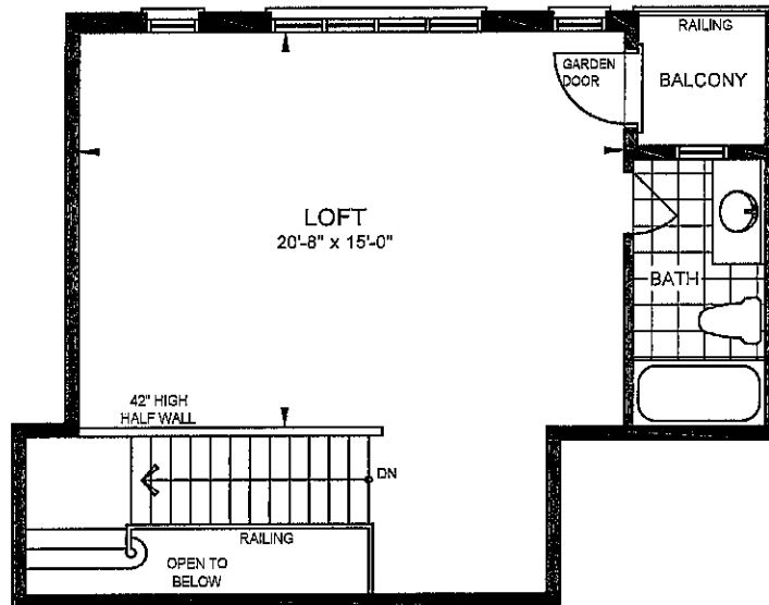
OPTIONAL LOFT PLAN ELEVATION 'A' & 'B'
